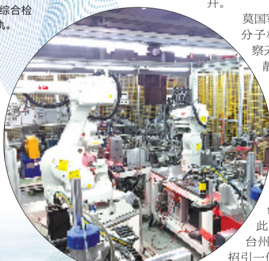
银轮股份智能化生产车间
