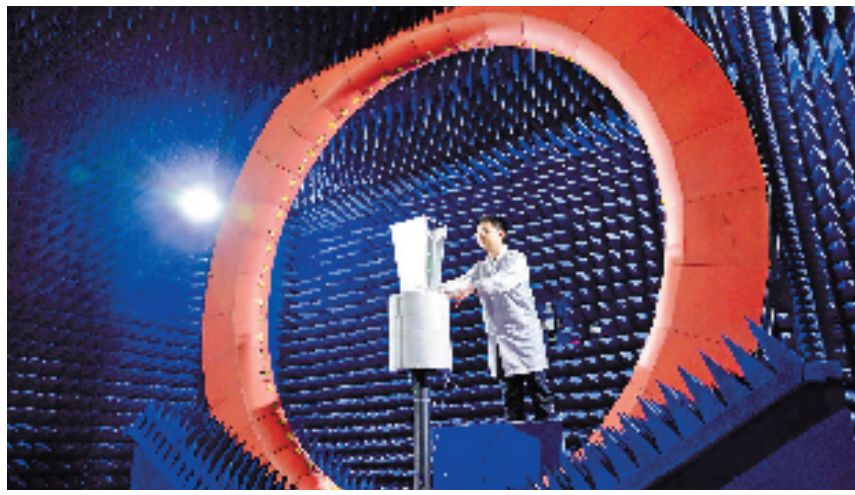
2024年4月27日,在位于湖州南太湖新区的电子科技大学长三角研究院,科研人员正在微波暗室实验平台开展测试工作。微波暗室实验平台是电子科技大学长三角研究院(湖州)的重大科研平台,主要为科研人员提供满足EMC测试要求的暗室环境(资料照片)。 本报记者 李震宇 摄
