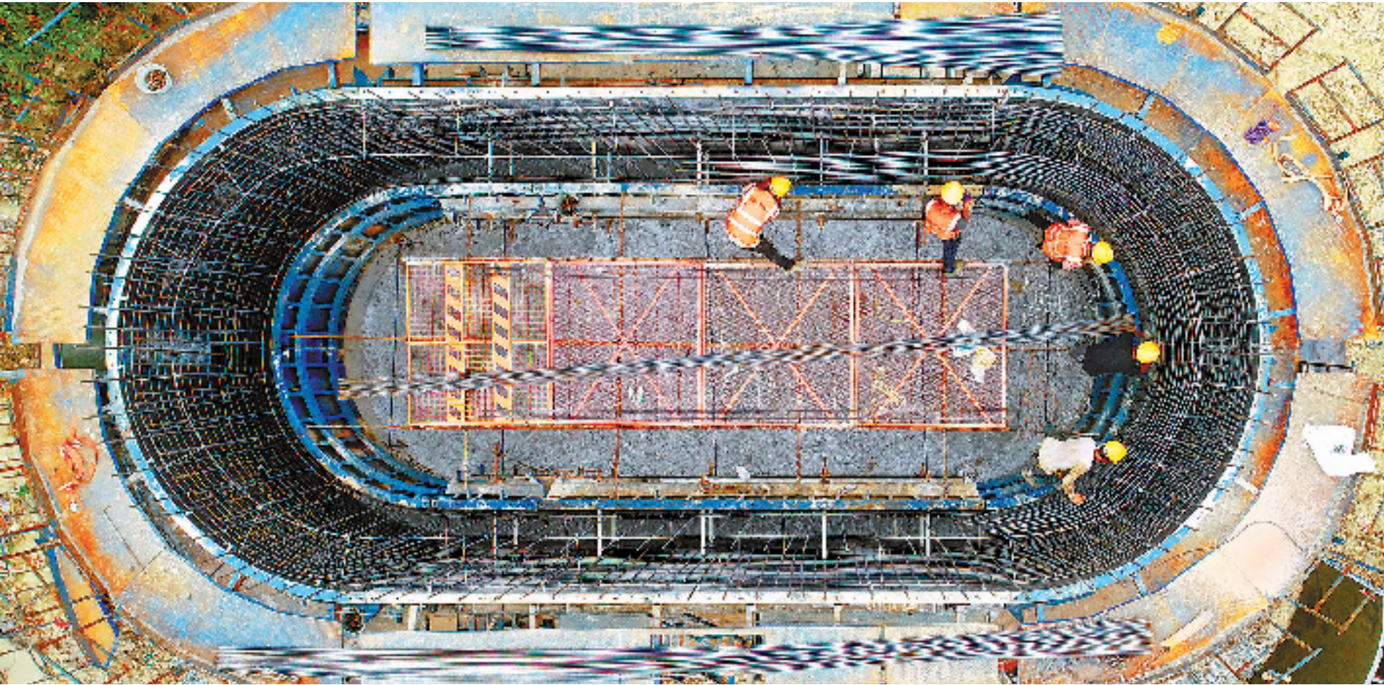
5月30日,浙江省杭绍台高铁线温岭至玉环铁路田岙大桥工程工地上,中铁十四局工人正在全力有序地推进最后4个桥墩的建设,力争在7月下旬26个桥墩全部建成。高铁线建成后,玉环至杭州仅需1个多小时。 拍友 吴达夫 摄
