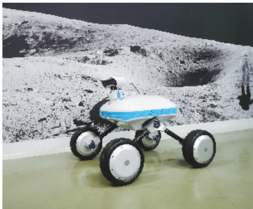
图为月面伴随机器人原理样机。
