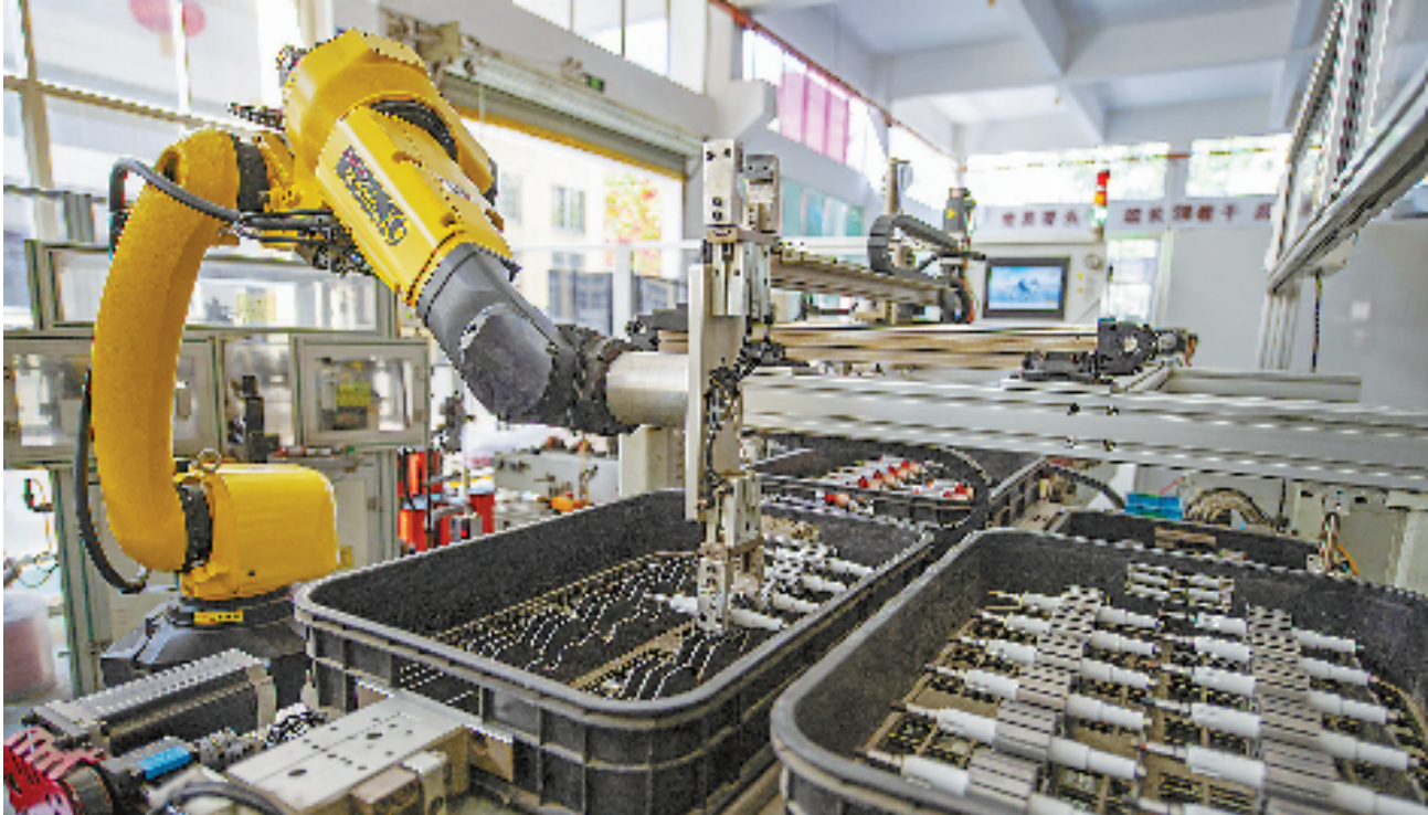
在永康市一企业自动生产线上,机器人手臂进行智能化生产。
