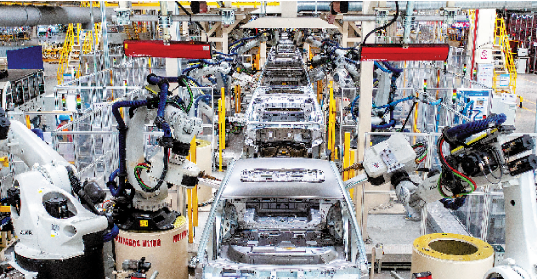
吉利汽车湖州长兴基地，全自动机器人正在高速运转。该基地是“5G+工业互联网”示范工厂，致力于提升数字化水平和科技创新能力。
