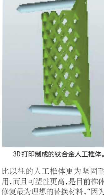
3D打印制成的钛合金人工椎体。
